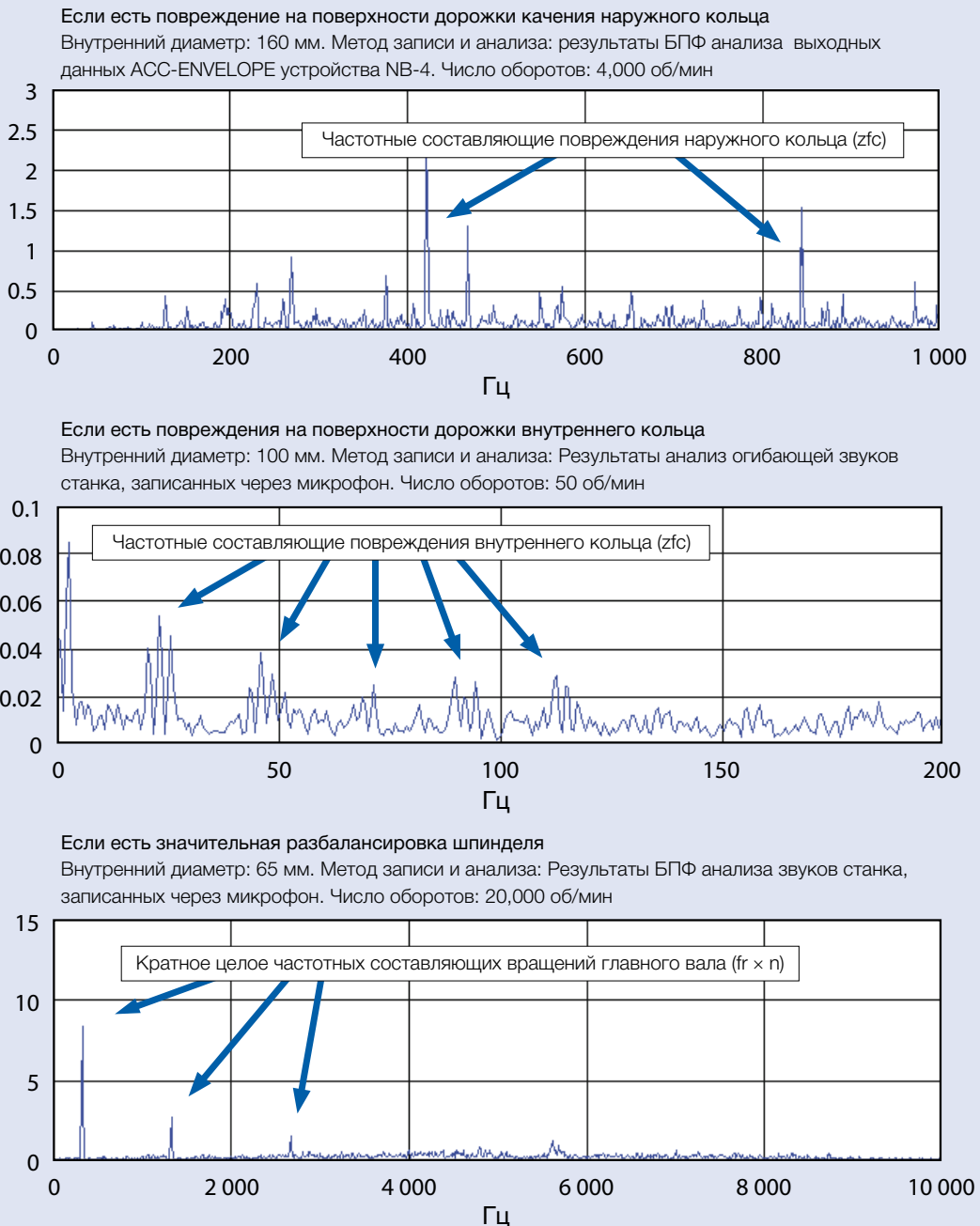
Рис. 2.4 Примеры результатов частотного анализа звуков и вибраций, проведенного при помощи программного обеспечения БПФ
